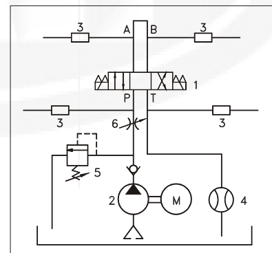
測試迴路
